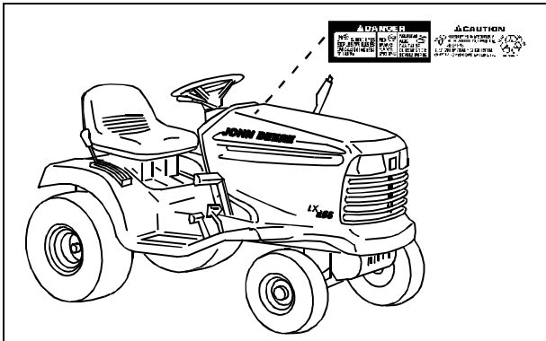
MIF M137060
