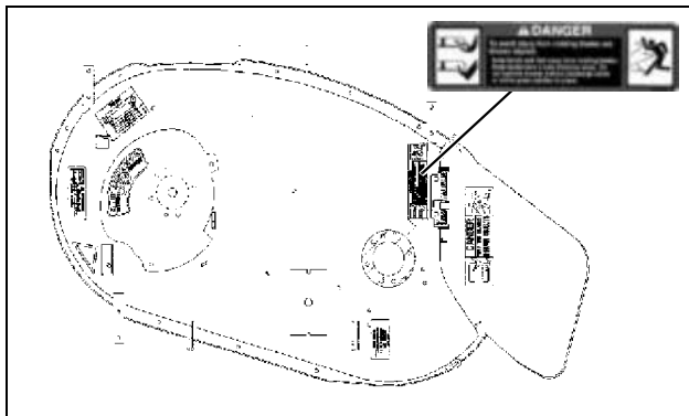
MX8380 M139128
